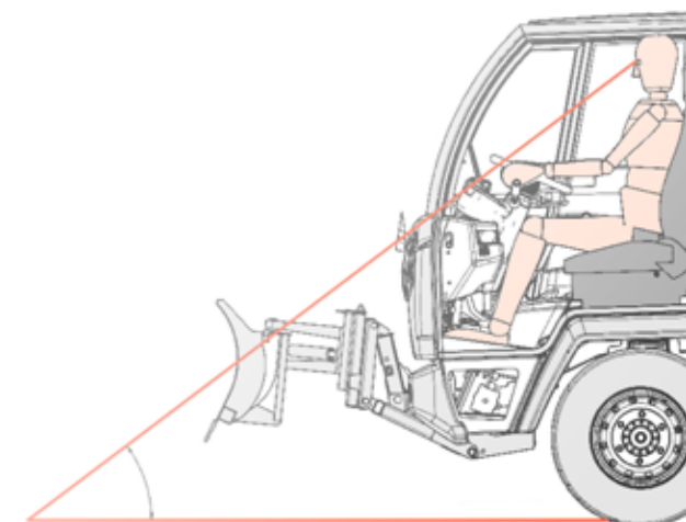
Mehr Raum, mehr Sicht, mehr Sicherheit: im ergonomisch designten Space-Frame-Fahrerhaus mit Panorama-Frontscheibe und integriertem Sonnenschutzbandfilter.
